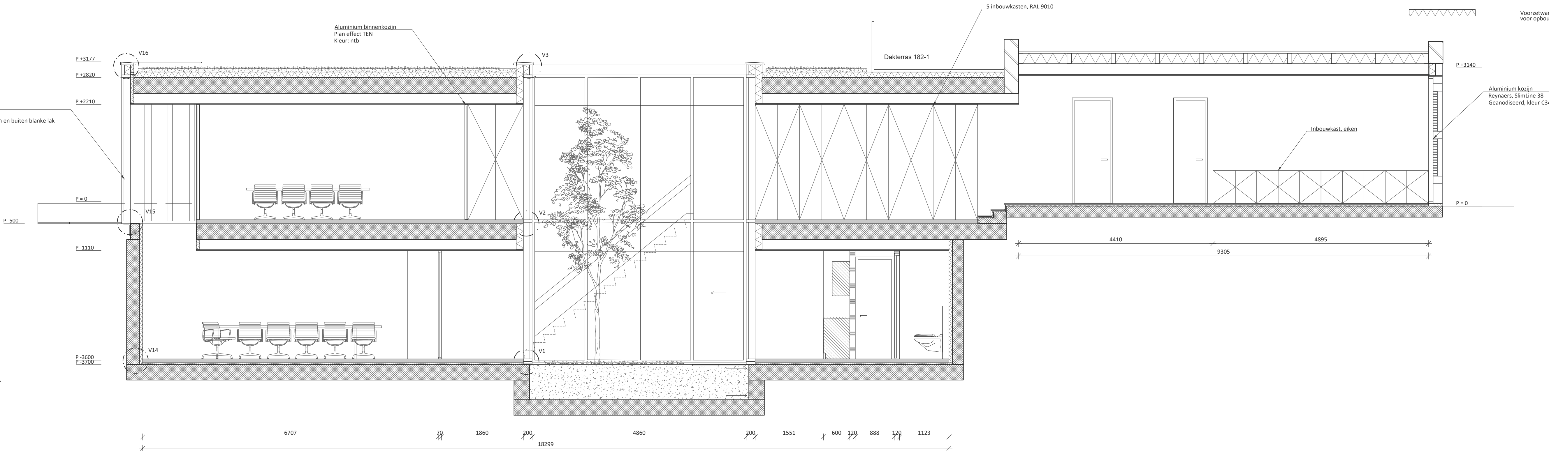
Doorsnede A
