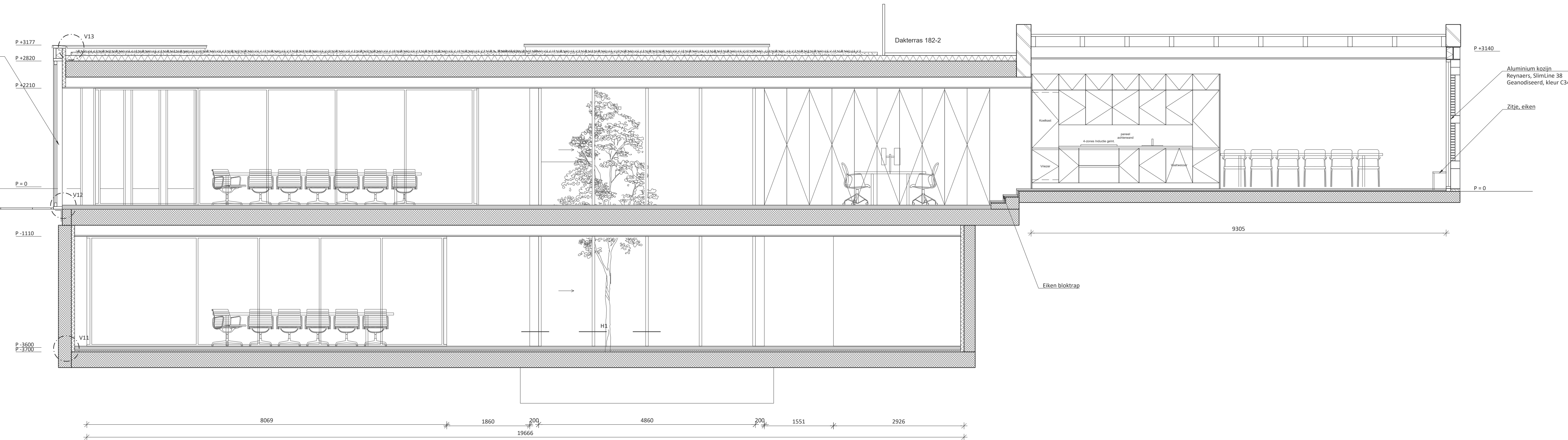
Doorsnede B
