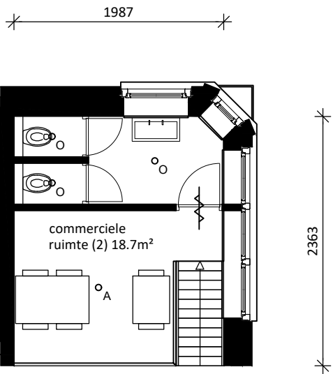
Eerste verdieping
