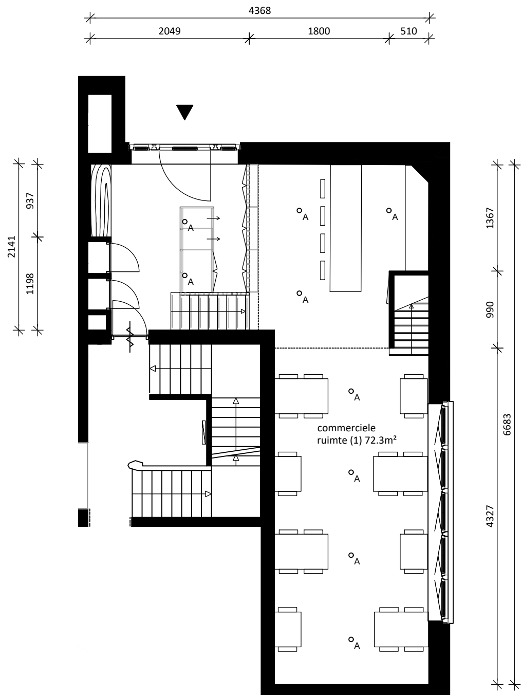
Begane grond
