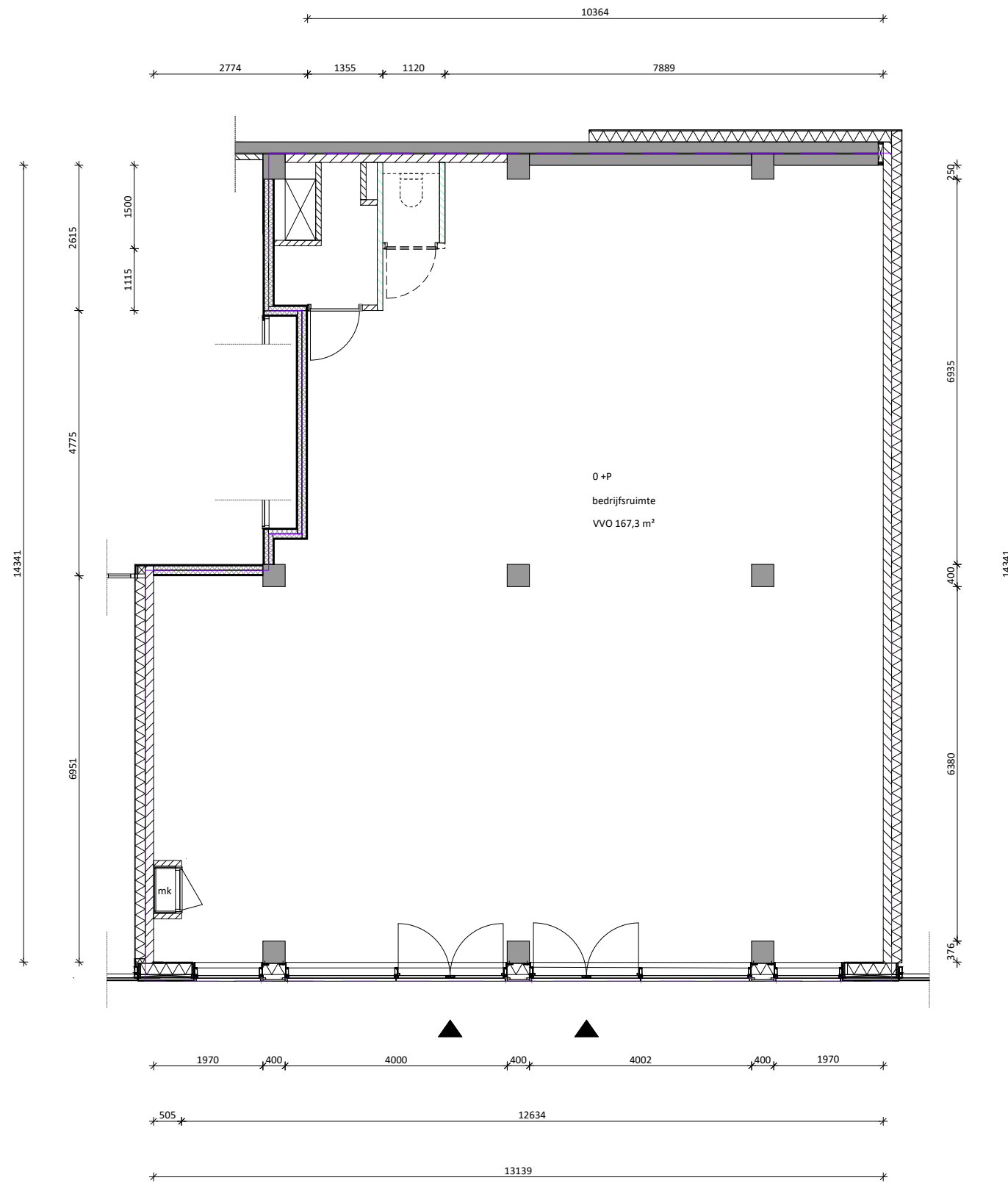
Begane grond
